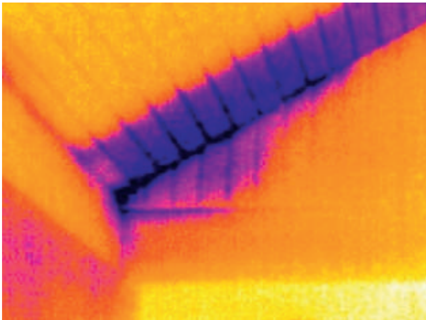
En kuldebro set gennem vores termografikamera
